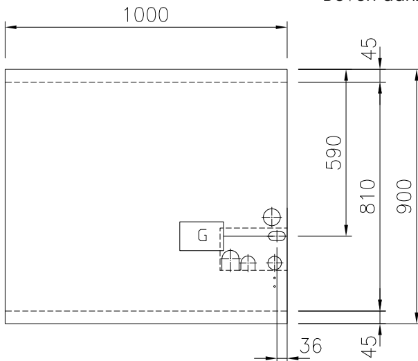
Boven aanzicht
