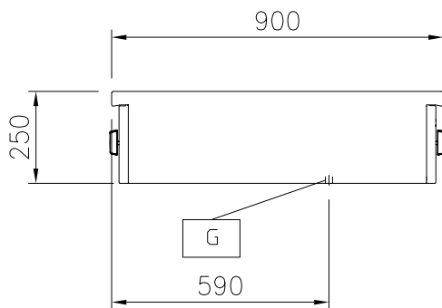
Zij aanzicht
